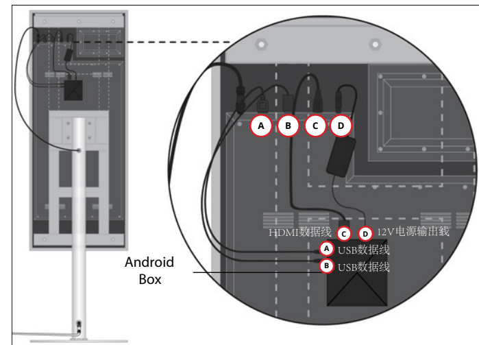
8 将以下数据线连接到安卓机顶盒：
