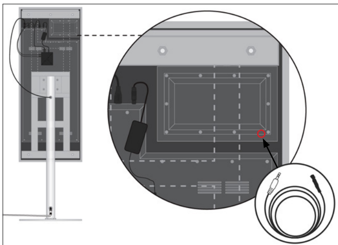
9 将1.5米的红外接收线的一端插在QAIO Flex的12.1”电视的背面，如上所示。
